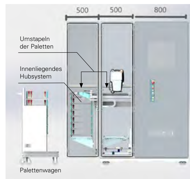
Modulare Zelle Schnittbild mit Palettierer
