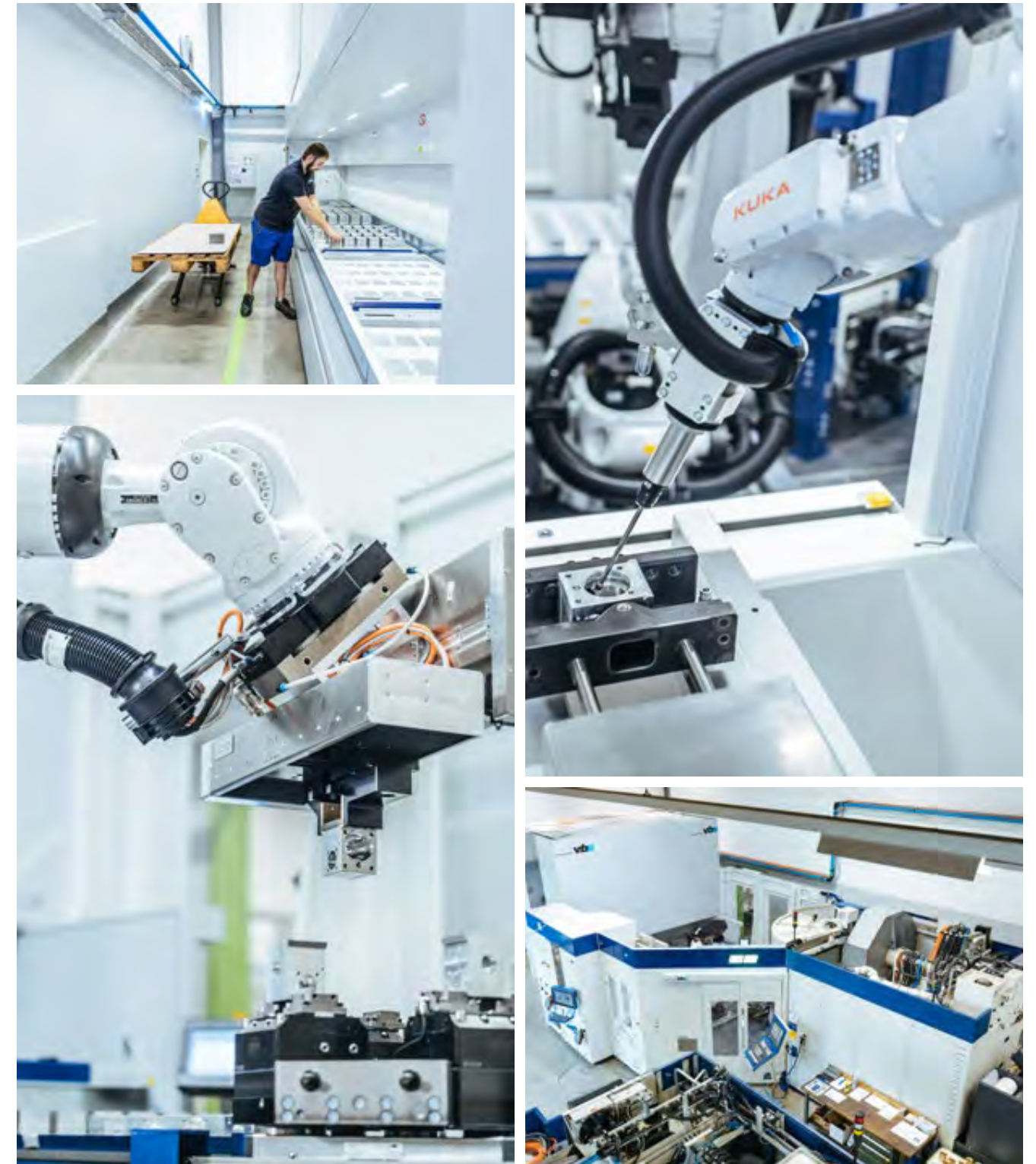
Praxisbeispiele VBA Roboterzelle mit Entgratstation
