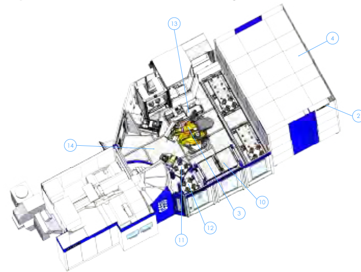
Layout Fräsmaschine KR 240 mit Entgratstation
