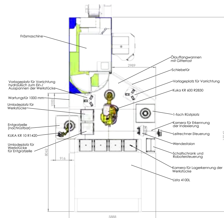
Layout Fräsmaschine KR 600 mit Wendestation
