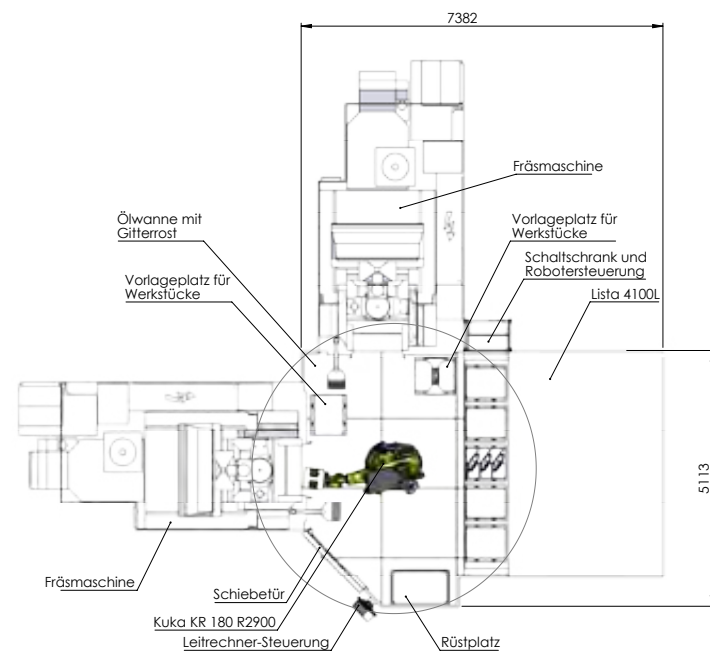
Layout Fräsmaschine KR 180 mit zwei Maschinen
