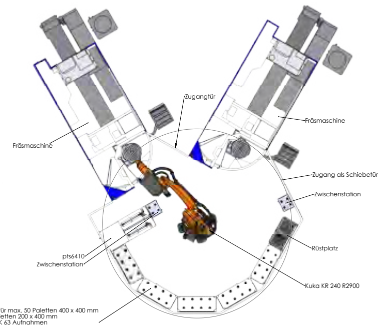
Layout Fräsmaschine KR 240 zwei Maschinen in V Stellung
