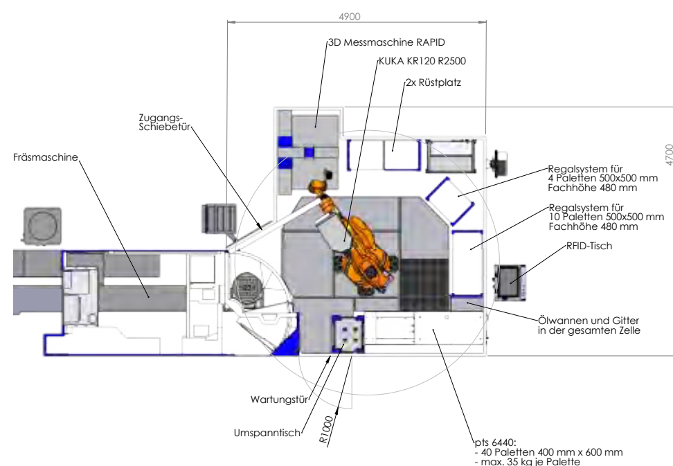
Layout Fräsmaschine KR120 mit Messmaschine
