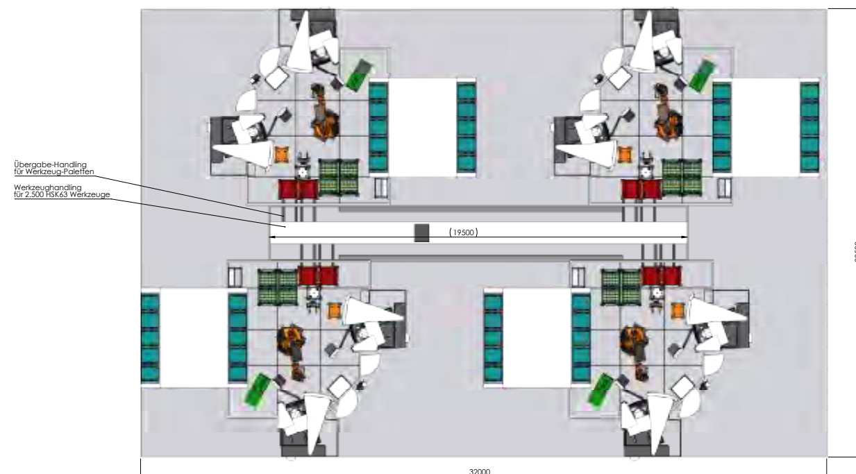
Layout Fräsmaschine KR240 mit 8 Maschinen und 2500er Werkzeugmagazin
