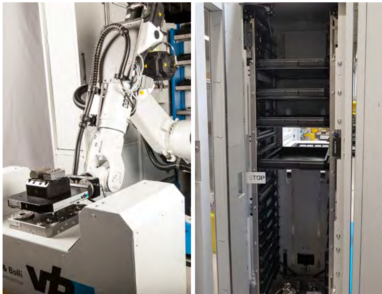
Praxisbilder VBA Roboterzelle Großanlage mit pts Werkstückpalettierer
