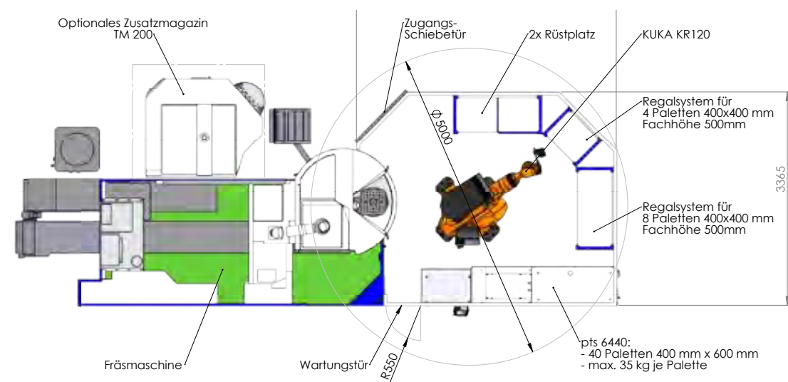
Layout Fräsmaschine KR120 mit pts
