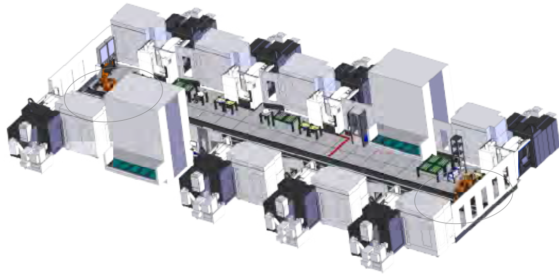
Layout Fräsmaschine KR 240 fahrbar mit 8 Maschinen
