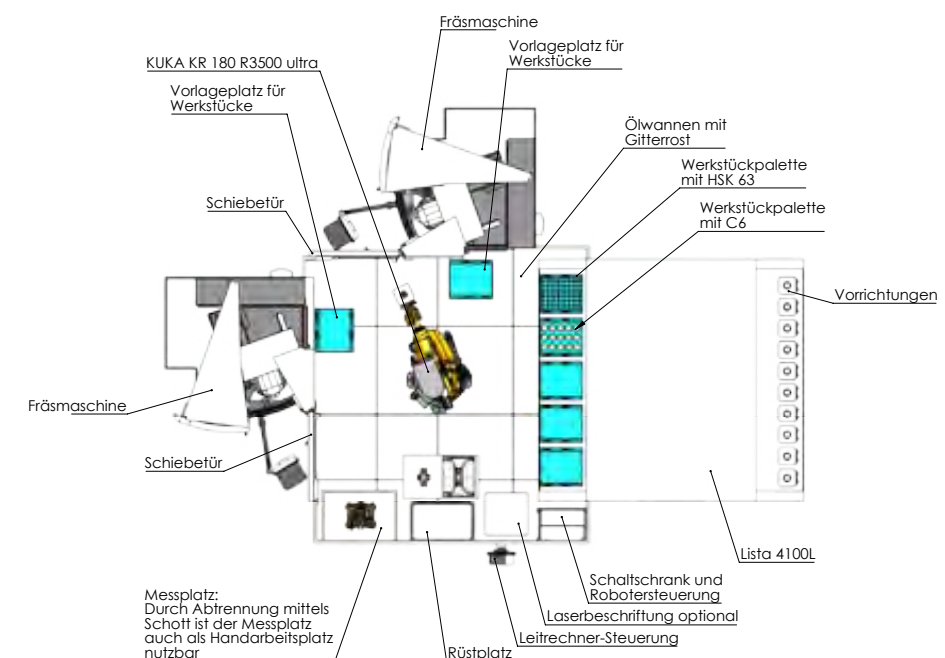
Layout Fräsmaschine KR 180 mit zwei Maschinen, Liftsystem und Messmaschine
