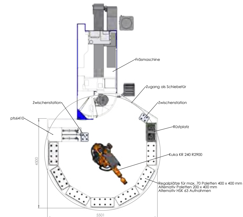
Layout Fräsmaschine mit 70 Palettenplätzen
