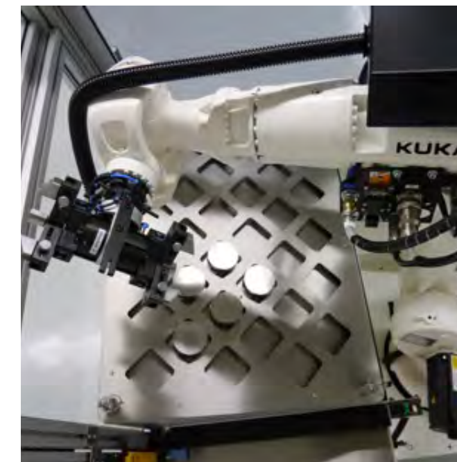
Mobile Roboterzelle mit Dreifachgreifer und Inlay
