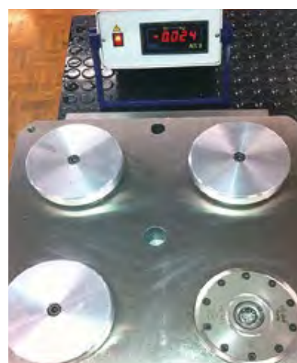
3 Kolben auf Spannstellung (1 Kolben in Fehlspannung) Hydraulik aus, drucklos, Restölinhalt ca. 24 cm 3
