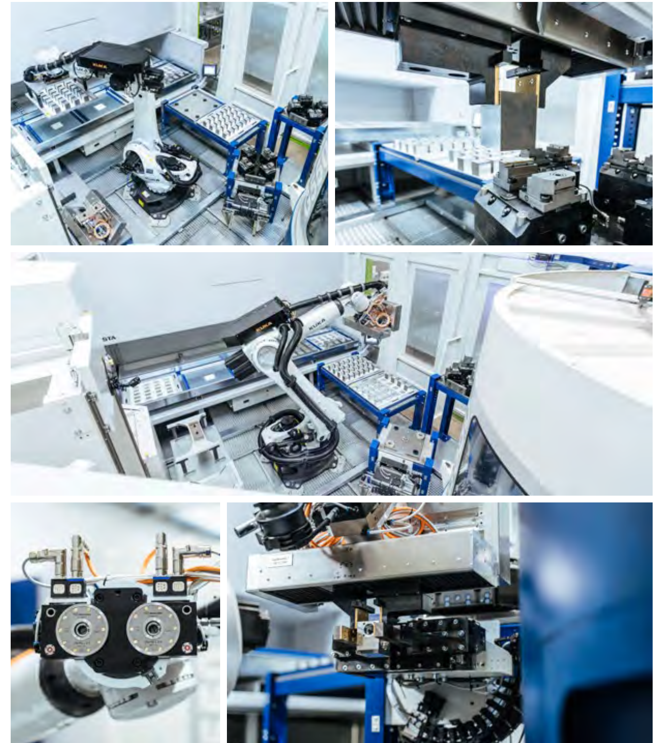
Praxisbilder VBA Roboterzelle Großanlage mit Liftsystem und Entgratzelle
