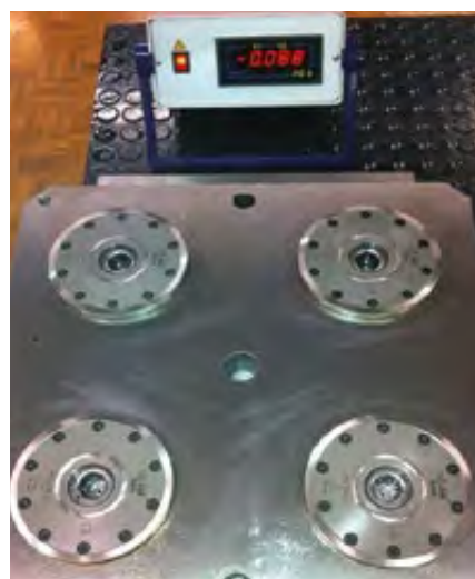
4 Kolben auf Lösestellung Hydraulik an, Restölinhalt ca. 88 cm 3
